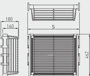
pełny wysuw / full extension / полное выдвижение
