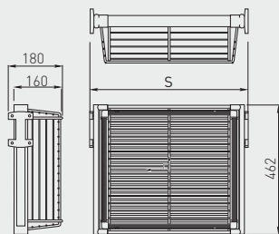
niepełny wysuw / partial extension / неполное выдвижение
